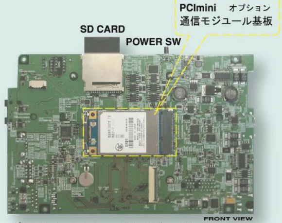
専用ベースキャリアボード
