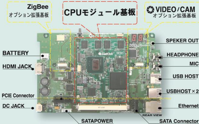
専用ベースキャリアボード
